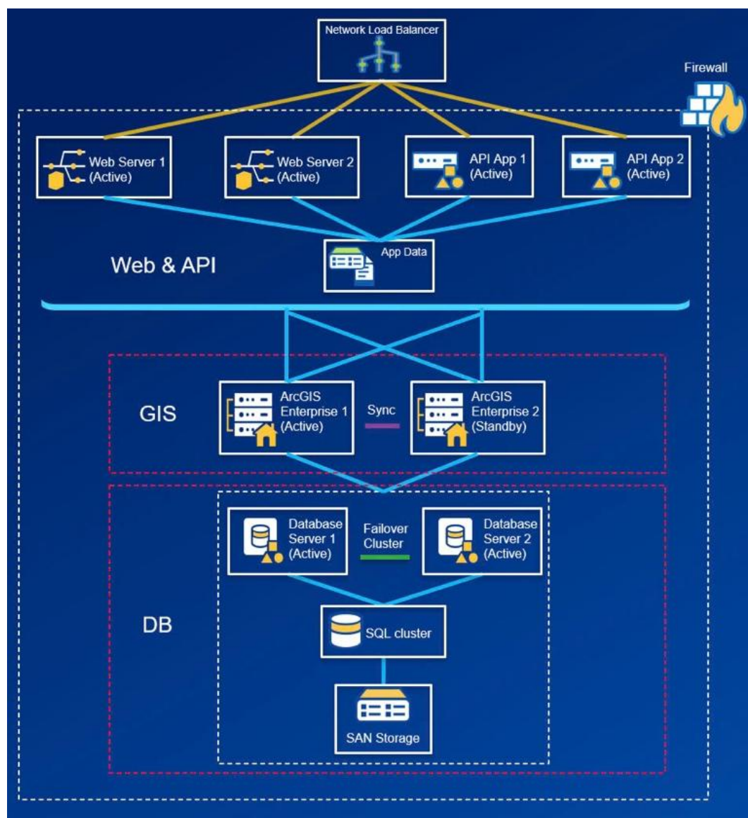
Mô hình triển khai máy chủ ảo
